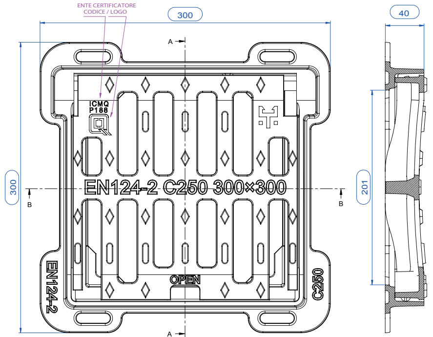
SEZIONE A-A
