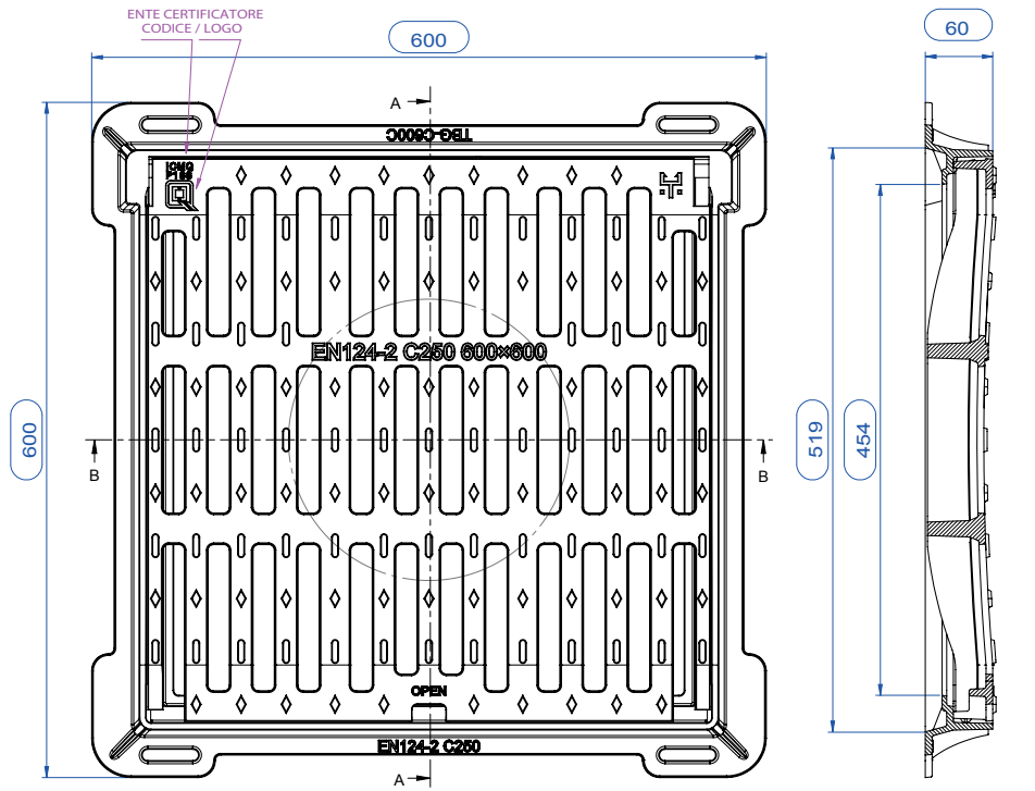
SEZIONE A-A
