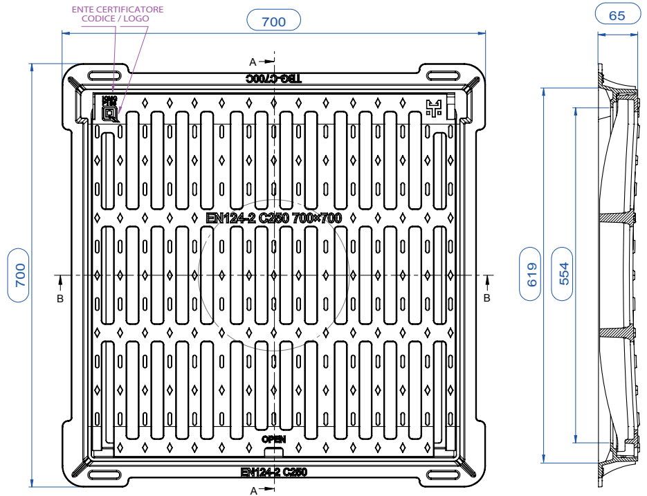
SEZIONE A-A
