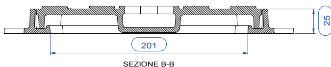
SEZIONE B-B
