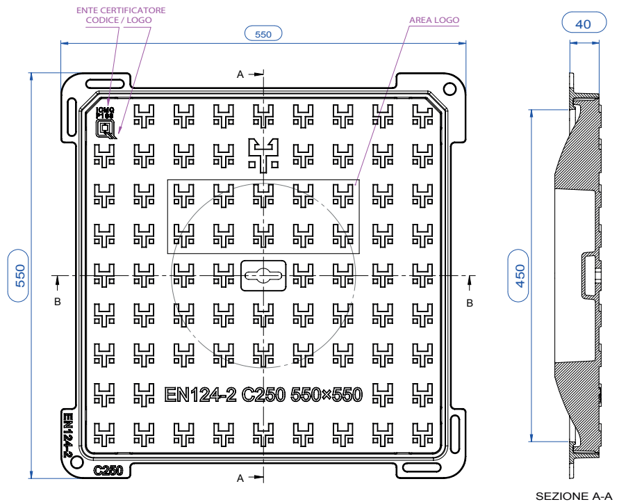
SEZIONE A-A
