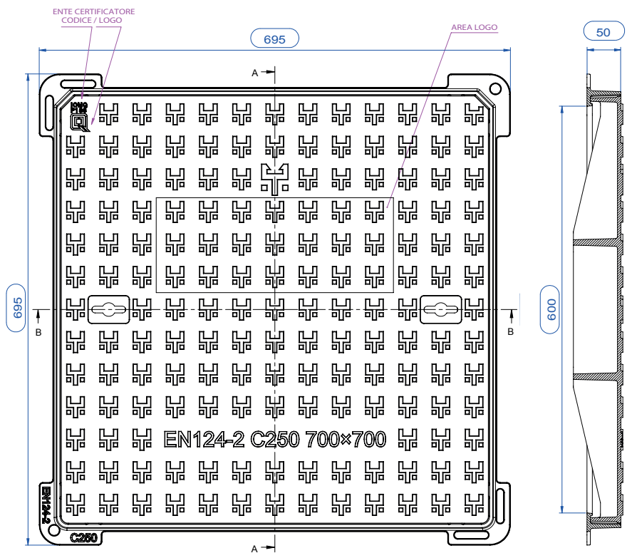
SEZIONE A-A
