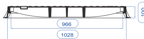
SEZIONE B-B
