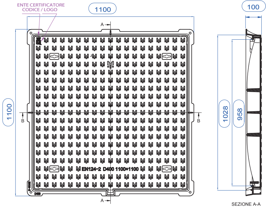
SEZIONE A-A
