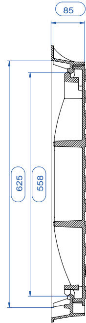
SEZIONE A-A
