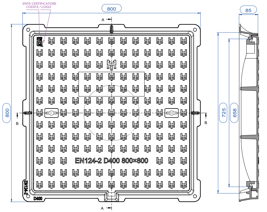
SEZIONE A-A
