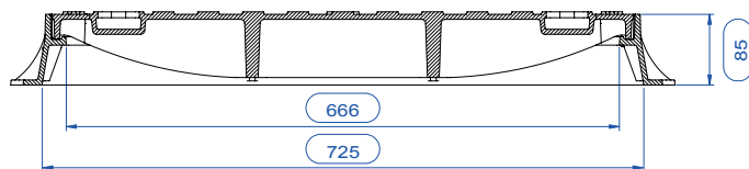
SEZIONE B-B
