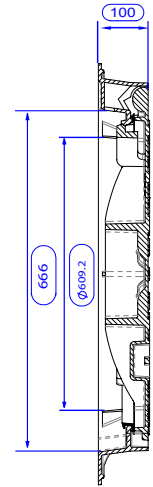
SEZIONE A-A
