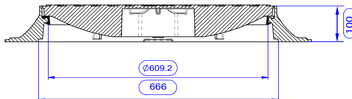
SEZIONE B-B
